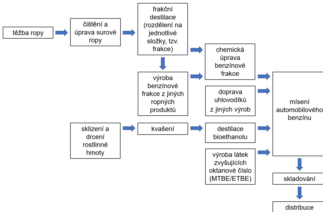
Schéma výroby automobilového benzínu
